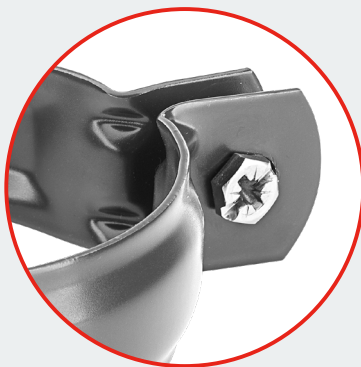
OBJÍMKA M10 NEREZOVÝ ŠROUB M6x20 (Pozink, Titan-zinek, Měď)
