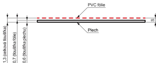
Struktura plechu:
