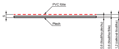
Struktura plechu:
